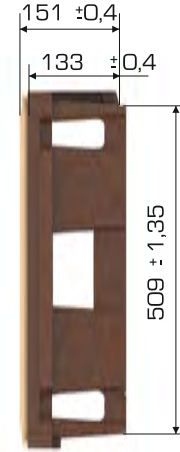
SECTION A-A
